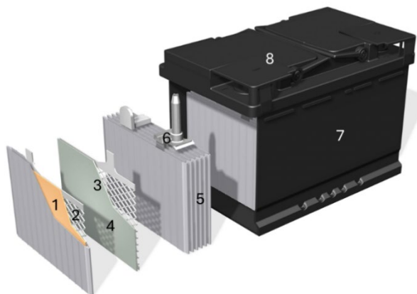
Figur 1 – Konceptuell design av ett LV Flooded blybatteri
