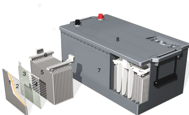
Figura 1 – Projeto conceptual de uma bateria CV de chumbo-ácido inundada
