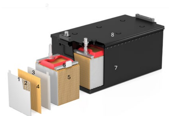
Figura 1 – Projeto conceptual de uma bateria CV de chumbo-ácido GEL - VRLA
