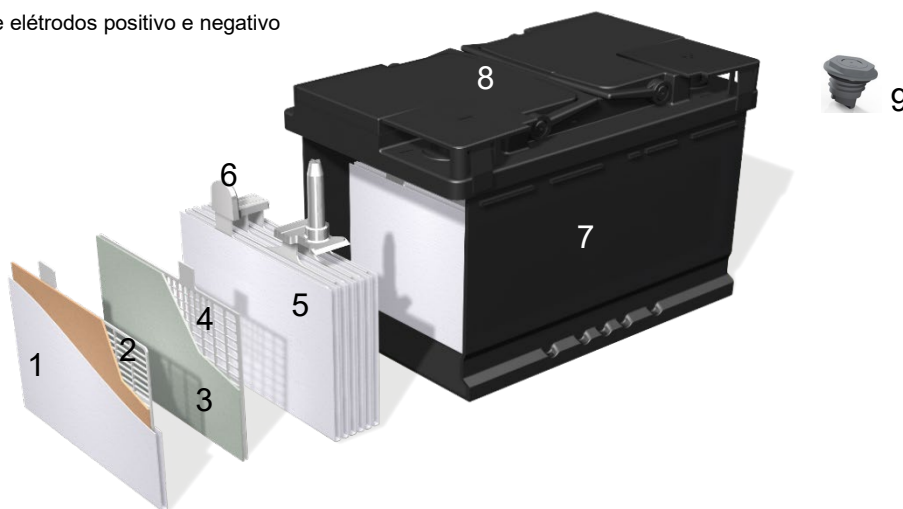
Figura 1 – Projeto conceptual de uma bateria prismática de chumbo-ácido AGM - VRLA
