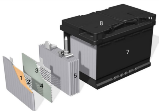
Figura 1 – Projeto conceptual de uma bateria de chumbo-ácido, inundada para veículos ligeiros
