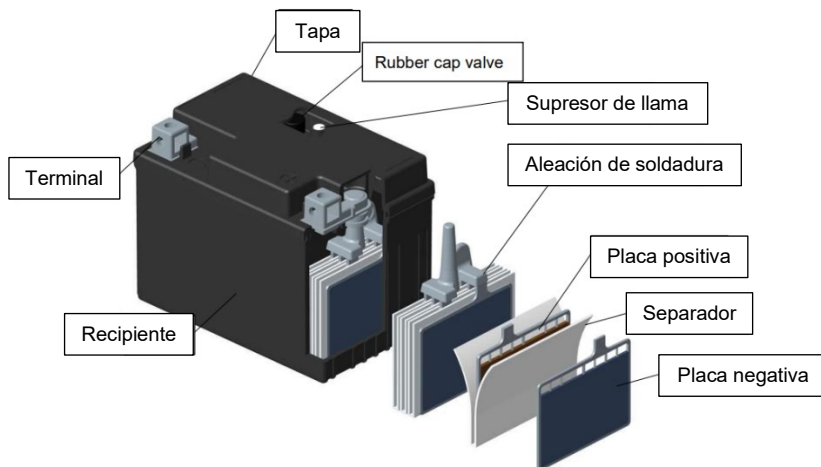
Figura 1 - Diseño conceptual de una batería de plomo-ácido Moto VRLA-AGM
