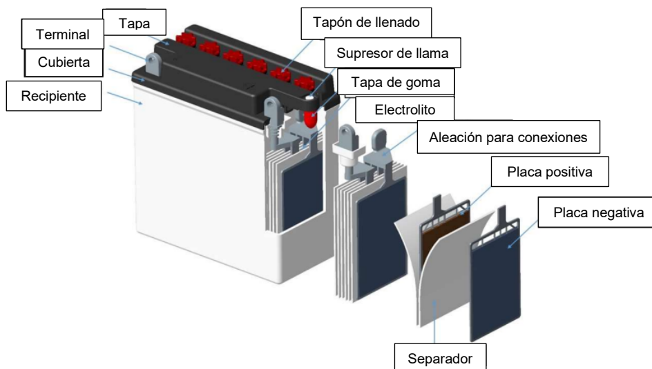
Figura 1 - Diseño conceptual de una batería de plomo-ácido MC inundada
