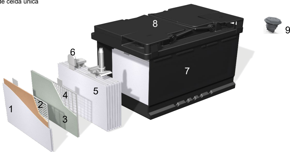
Figura 1 - Diseño conceptual de una batería prismática de plomo-ácido VRLA-AGM
