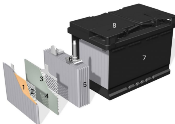
Figura 1 – Diseño conceptual de una batería de plomo-ácido inundada para turismos
