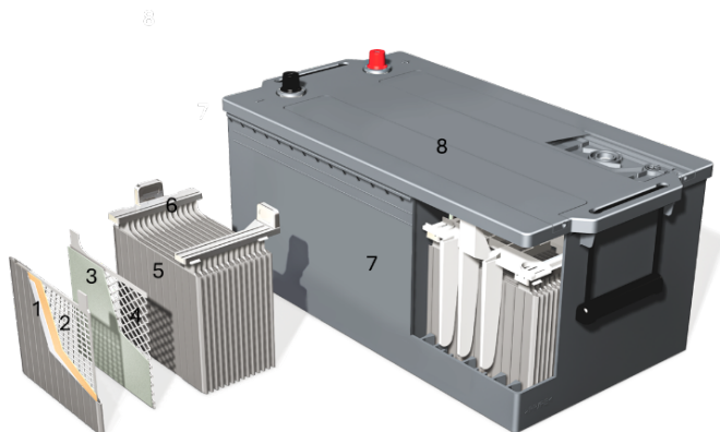
Obrázek 1 – Konceptní návrh konstrukce olověné baterie s kapalným elektrolytem a s konstantním napětím
