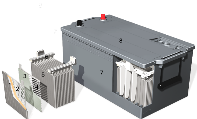
Joonis 1 – Veoki sukeldatud pliihappeaku kontseptuaalne disain
