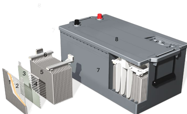
Kuva 1 – CV Flooded -lyijyakun konseptisuunnittelu
