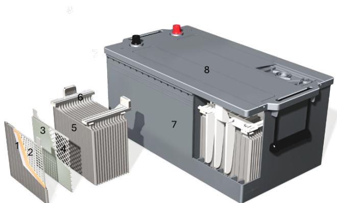
Σχήμα 1 - Εννοιολογικός σχεδιασμός μπαταρίας μολύβδου-οξέος υγρού ηλεκτρολύτη CV
