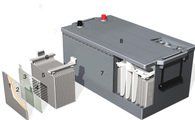
1. ábra – Tehergépjárművekhez használható folyadékos típusú ólom-sav akkumulátor koncepcionális terve
