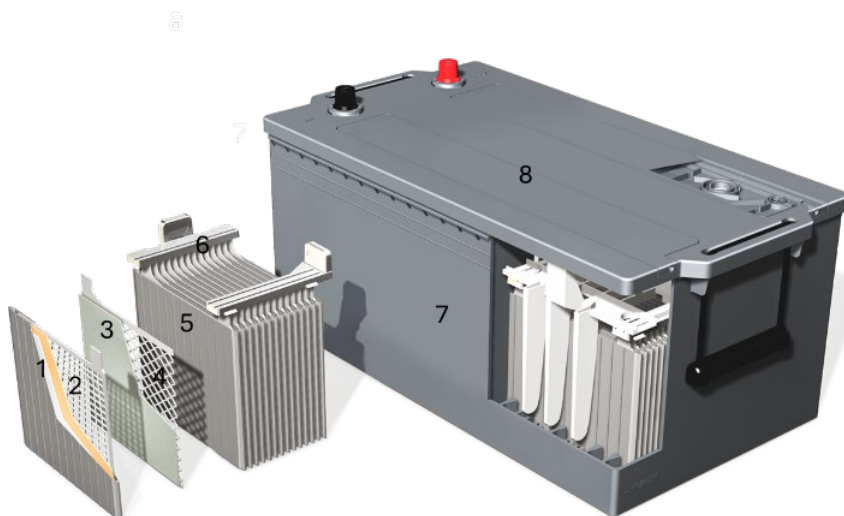
Figura 1 - Progetto concettuale di una batteria CV al piombo acido libero
