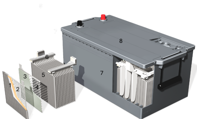
1 iliustracija. CV užtvindyto švino rūgšties akumuliatoriaus koncepcinis dizainas
