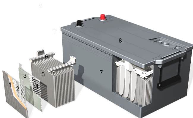
1. attēls. Tehnoloģijas CV Flooded svina-skābes akumulatora konstrukcijas meti
