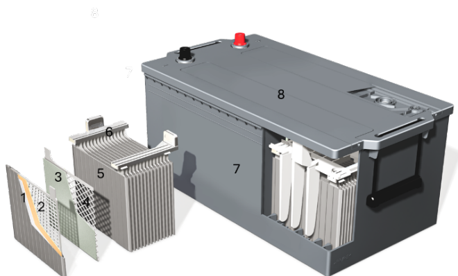
Figura 1 – Disinn kunċettwali ta' batterija tač-čomb u l-ačidu CV li fiha Elettroliti Likwidi (Flooded)
