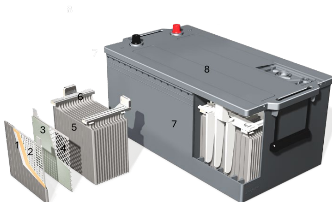
Figuur 1 – Conceptueel ontwerp van een CV-loodzuuraccu
