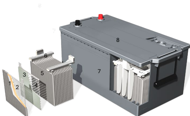
Figur 1 – Konceptuell design av ett CV Flooded blybatteri
