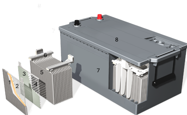
Slika 1 – idejna zasnova mokrega svinčevega akumulatorja CV
