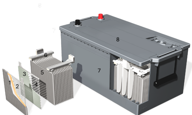
Slika 1. – Koncept dizajna olovno-kiselinske baterije s tekućim elektrolitom sa stalnim naponom (CV)
