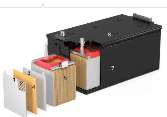
Obrázek 1 – Konceptní návrh konstrukce olověné baterie GEL-VRLA s konstantním napětím
