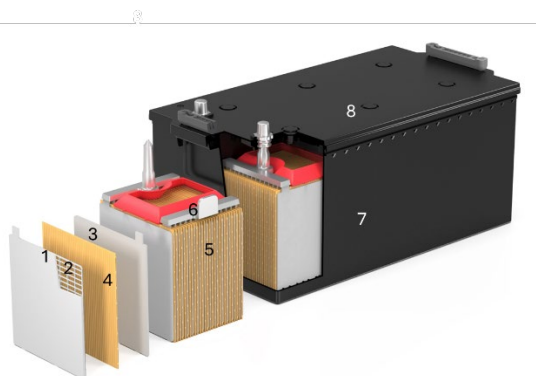
Abbildung 1 – Aufbau einer Blei-Säure-GEL-VRLA-Batterie für Nutzfahrzeuge
