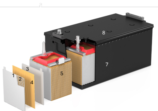
Slika 1 – Koncept dizajna olovno-kiselinske baterije sa stalnim naponom (CV) GEL-VRLA
