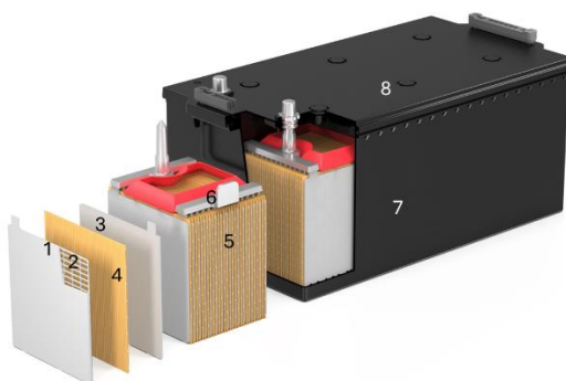
Fíor 1 - Dearadh coincheapúil ceallraí aigéad luaidhe CV GEL-VRLA
