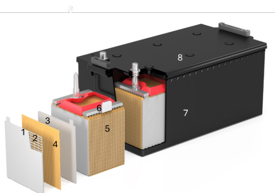
1 iliustracija. CV GELINIO-VRLA švino rūgšties akumuliatoriaus koncepcinis dizainas
