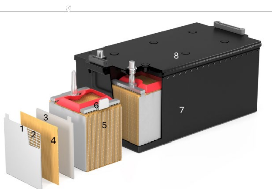
Figuur 1 – Conceptueel ontwerp van een CV GEL-VRLA loodzuuraccu
